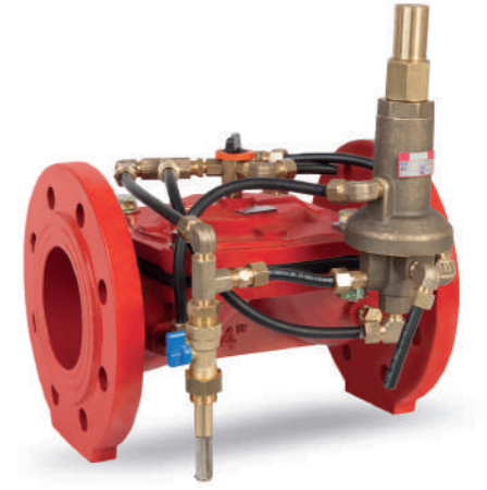
Debi Kontrol Vanası Flow Control Valve
